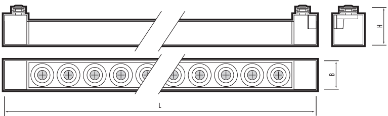
Рис.1 Прожектор PTR 44
